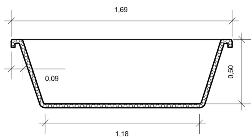
Corte BB
